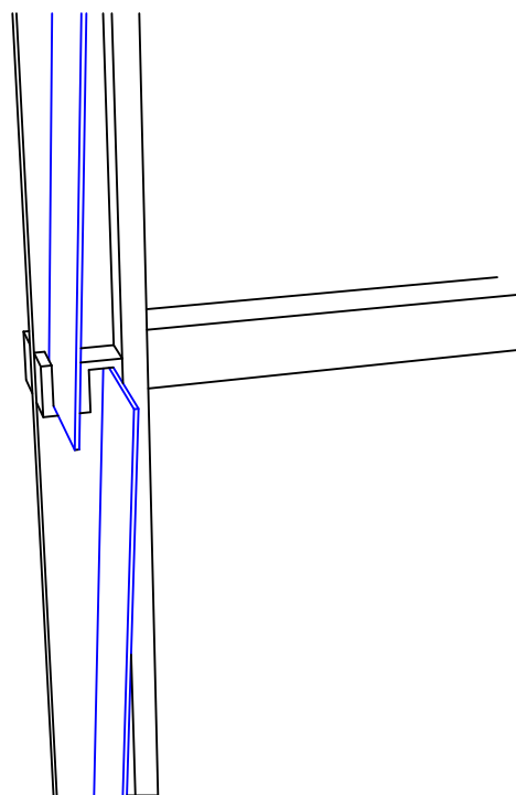
• DETAIL UCHYCENÍ
