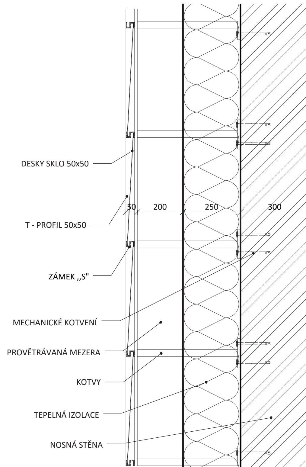
• ŘEZ FASÁDOU
