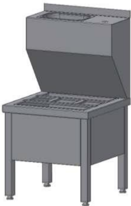
Kombinovaná výlevka s rámem a umyvadlem
