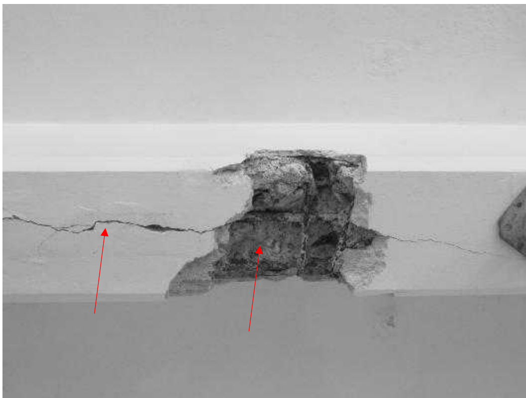
Foto 14: Hlavní budova 1.NP, místnost M2: trhliny na spodním líci středu tránu cca 3až4 mm. Trhliny oddělují krycí vrstvu betonu od výztuže, beton samovolně vypadává, povrchová koroze výztuže.
