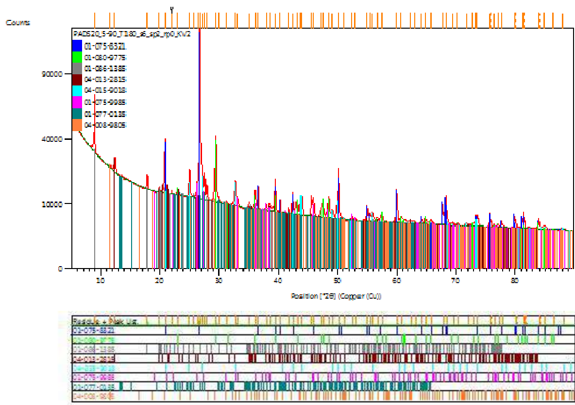
Obr. 2: Rentgenový práškový difraktogram vzorku betonu KV2
