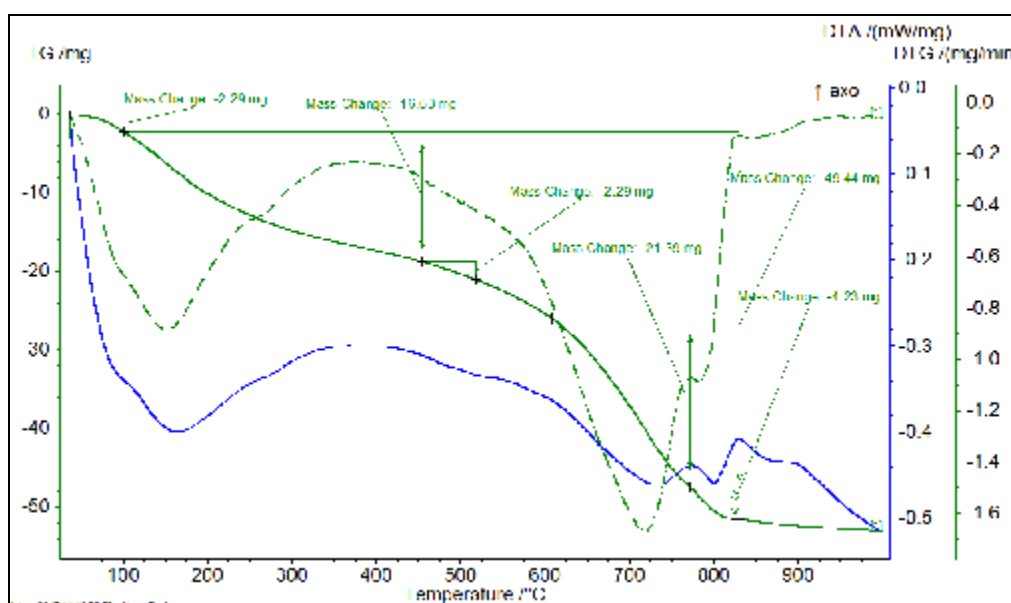
Obr. 3 Záznam termické analýzy vzorku V1.2
